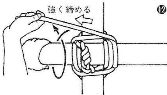
巻き結びを行う(12-14)
