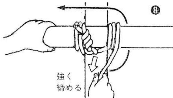
2-3回縦方向に巻きつけたら、横の柱の後ろを通して、縦の柱の前に横方向にロープを回す(これを“割り”という)
