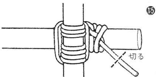
(裏側から見た完成図)
