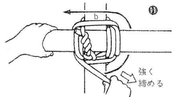
8と同様に“割り”を入れる。このとき、b部の“巻き”の内側にロープを回すこと。“割り”は3回ぐらい行う
